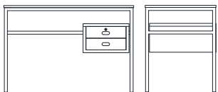
Escritorio 2 cajones. 110 x 60 x 75
